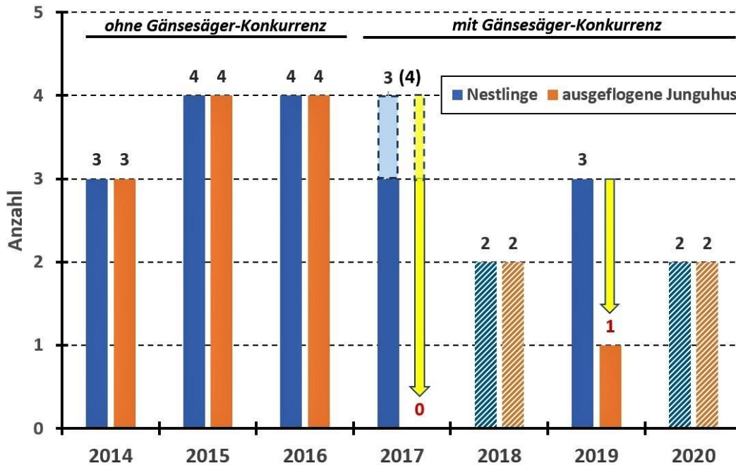
Abb. 16. Reproduktion der Uhus 2014-20 in der Lösshöhle (gefüllte Säulen) und an einem Ausweichbrutplatz (schraffiert) unter dem Einfluss von Brutplatzkonkurrenz durch Gänsesäger; Pfeile markieren den Verlust von Nestlingen. – Eagle Owl reproduction 2014-20 in the loess cavity (solid columns, blue = number of nestlings, orange = number of fledged young) and at an alternative nesting site (hatched columns) as affected by nest site competition from Goosanders; arrows indicate loss of nestlings.
